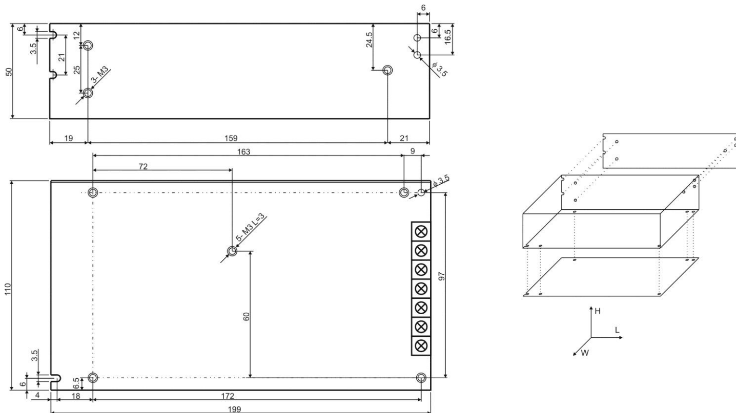
Rysunek 2. Widok mechaniczny zasilacza.
